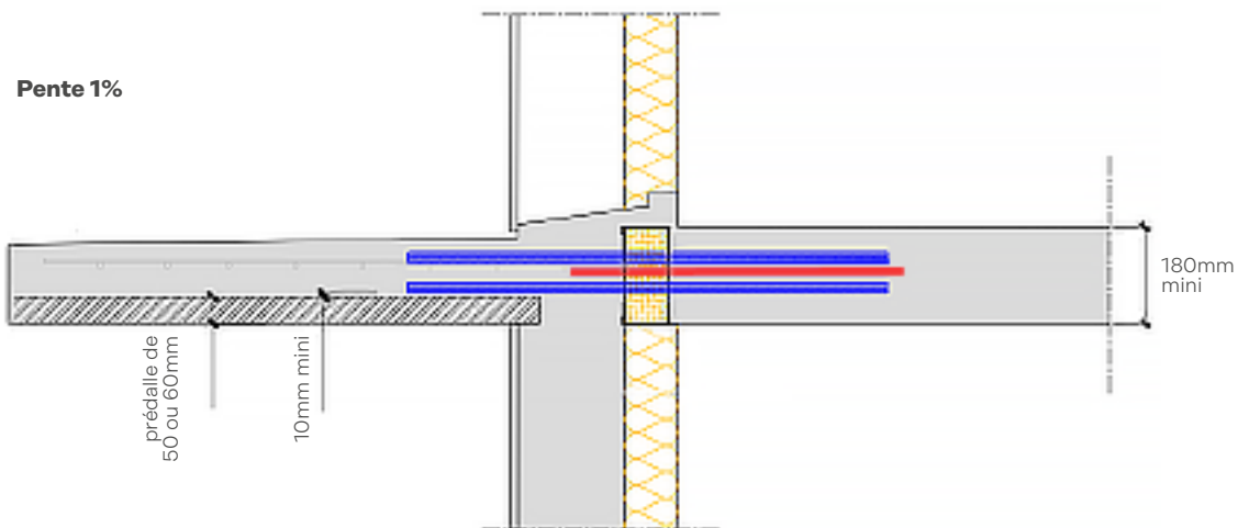
Application HIB avec prédalle BA ou précontrainte côté balcon
