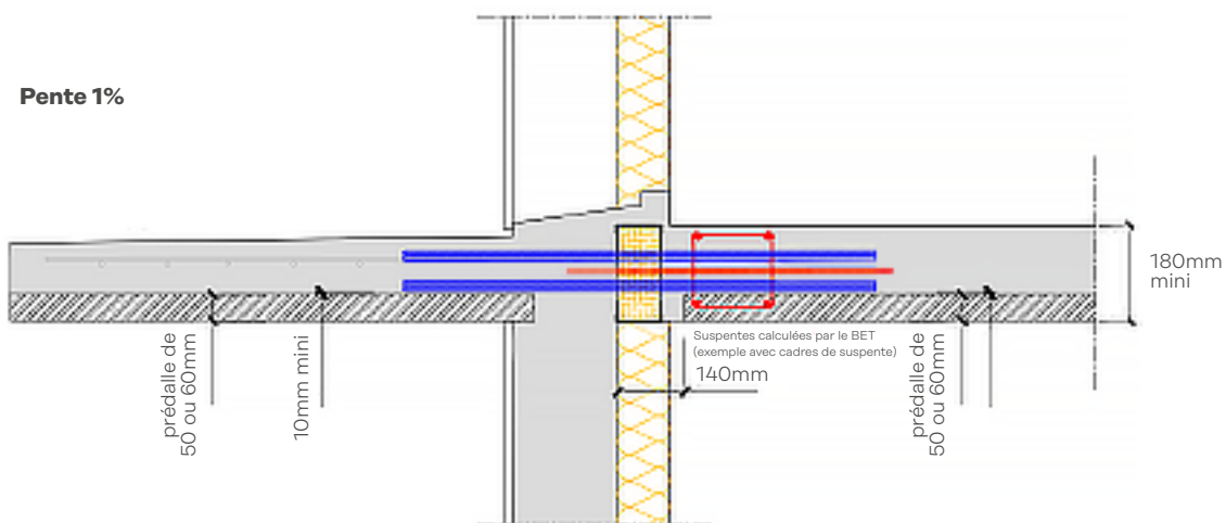
Application HIB avec prédalles BA ou précontraintes de chaque côté
