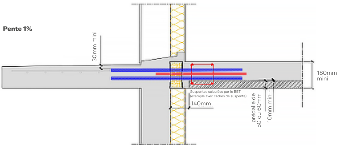
Application HIB avec prédalle BA ou précontrainte côté dalle intérieure
